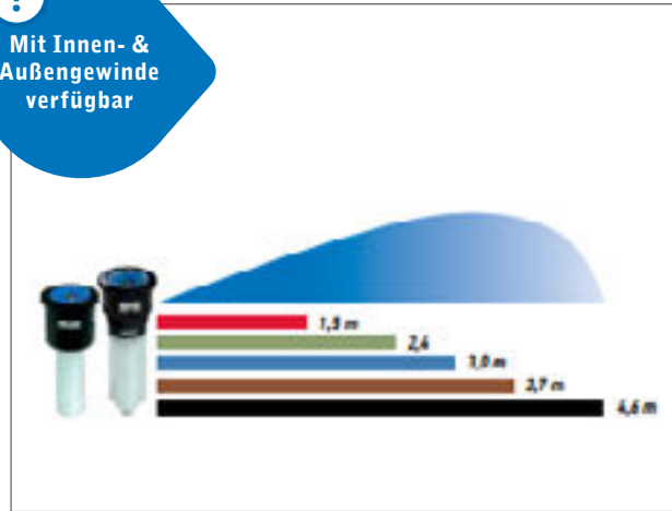
Sprühdüse „Precision“ Statisch, verschiedene Wurfweiten und Sektoren
